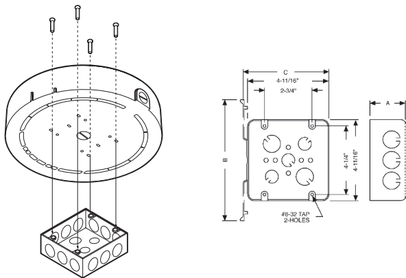
Type A: Handy boxes
